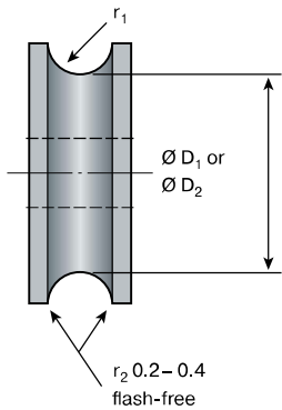
Fig. 2.21 Pulley gland radius
